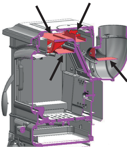
2 - DÉFLECTEUR DE FUMÉE
