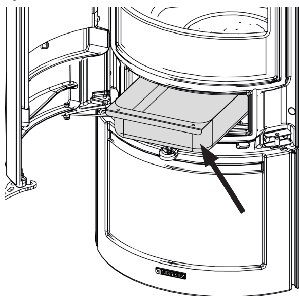
1 - TIROIR DE COLLECTE DES CENDRES
